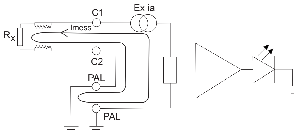
Fig. 13: Schéma fonctionnel du système de contrôle de mise à la terre TERRALIGHT
