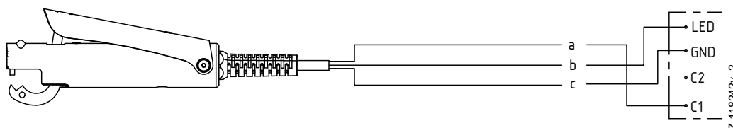
Fig. 12: Exemple de connexion d'un contacteur de mise à la terre TERRALIGHT avec LED d'état intégrée
