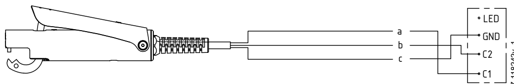
Fig. 11: Exemple de connexion d'un contacteur de mise à la terre TERRALIGHT
