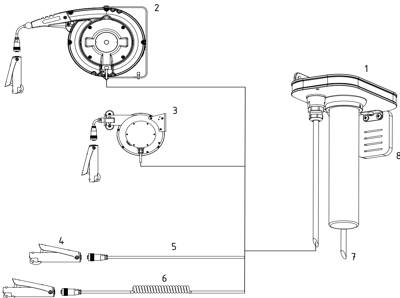
Fig. 1: Vue d'ensemble du système de contrôle de mise à la terre TERRALIGHT
