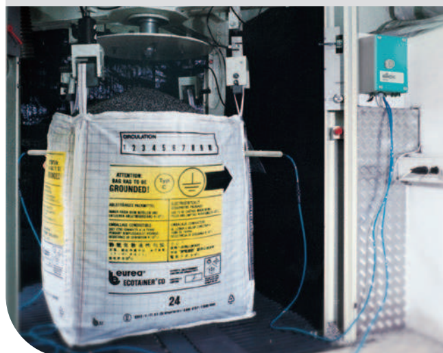
Protection de BIG-BAG durant le remplissage
