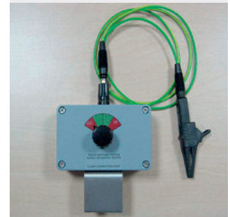
Testeur TCT pour contrôler le bon fonctionnement du système de mise à la terre TERRACAP TCB040
