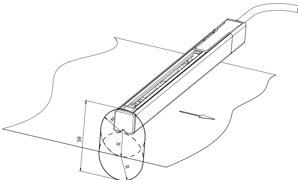
Fig. 3 : Zone sans matériaux conducteurs reliés à la terre avec les dimensions R
