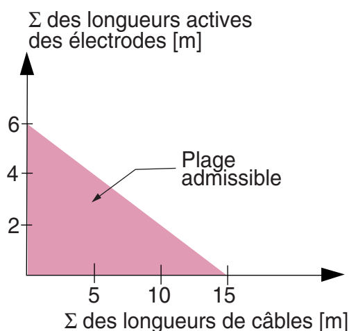
Fig. 4 : Charge possible de l'alimentation ES47 en fonction de la longueur active de l'électrode et de la longueur totale du câble de haute tension
