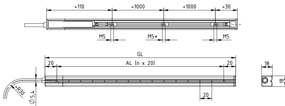
Fig. 2 : Montage de l'électrode de décharge R47
