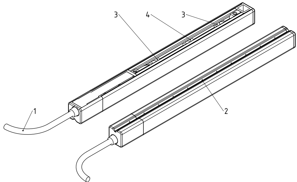
Fig. 1 : Vue d'ensemble de l'électrode de décharge R47
