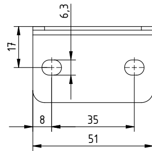
Fig. 12: Équiere de fixation
