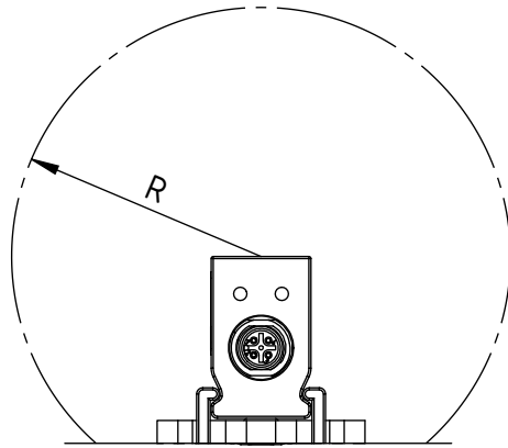
Fig. 7: Zone exempte de matériau conducteur, reliés à la terre autour de l'électrode de décharge
