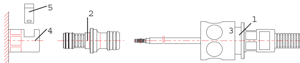
Fig. 11: Fiche de connexion rapide pour composants de charge
