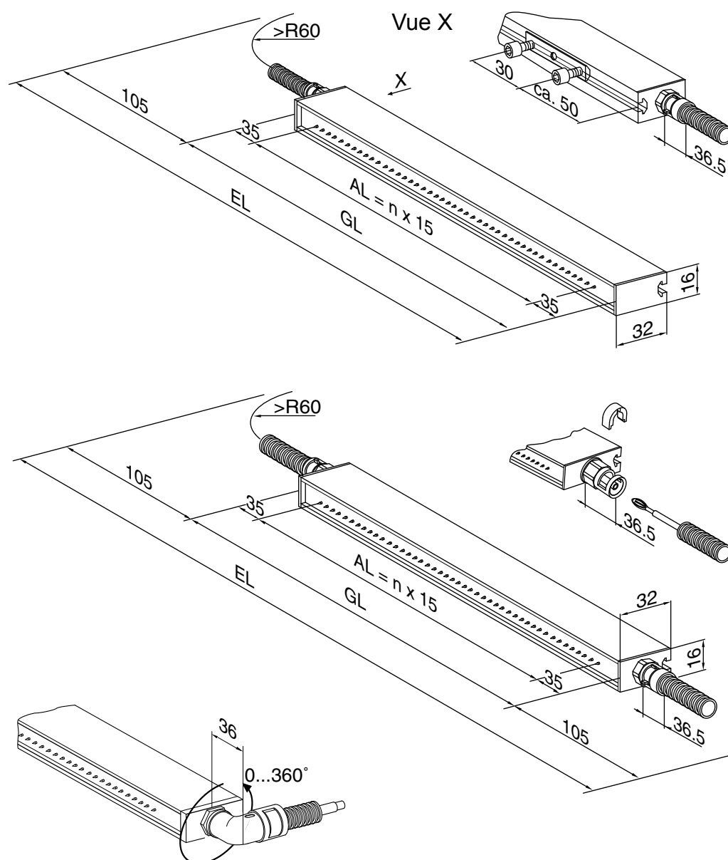
Fig. 10: Dimensions de l'électrode de charge, variantes de branchement du câble de haute tension
